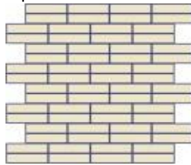
Dubbel halfsteens
